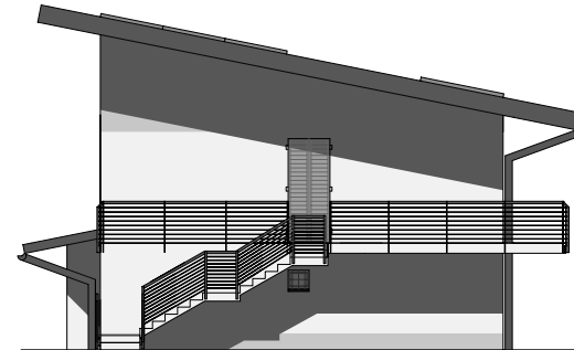
PROSPETTO NORD-EST
