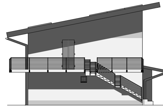
PROSPETTO SUD-OVEST
